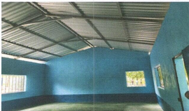
Foto 3: Sustitucion de estructura de soporte de madera, por metal
