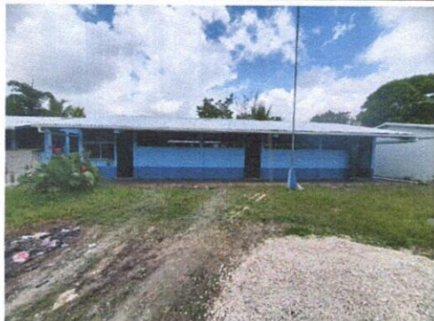
Foto: 1 SUSTITUCIÓN DE LÁMINA POR LÁMINA TROQUELADA ALUZING CALIBRE 26
