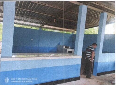
Foto 5: Pintura en muros exteriores e interiores
