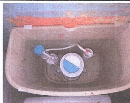
Foto 6: uestitucion de accesorios inodoro(contrallave,tubo de abasto y tanque
