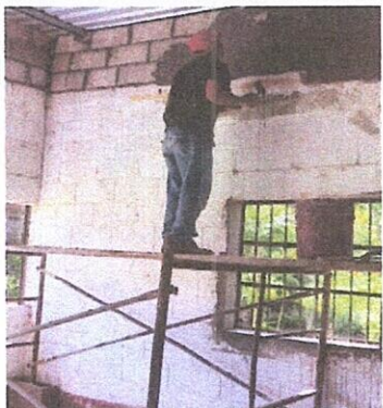
Foto11: Repello en muro
