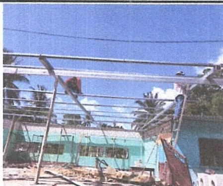
Foto 2: Sustitución de estructura de soporte
