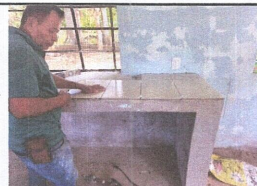
Foto 12: Instalacion de azulejo en estufa rural
