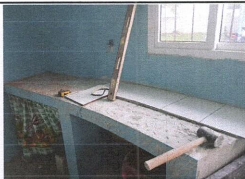
Foto 5: Instalación de azulejo en estufa rural
