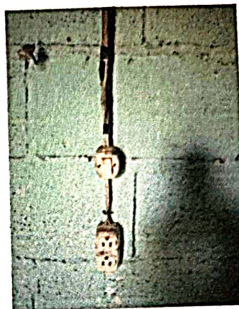
Foto 3.6: Instalación de unidades fuerza (tomacorriente), incluye cable eléctrico
