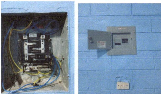
Foto 5: Reparación de sistema eléctrico: sustitución de lámparas, plafoneras, interruptores, tomacorrientes, sustitución de ducto eléctrico y reparación de cable eléctrico
