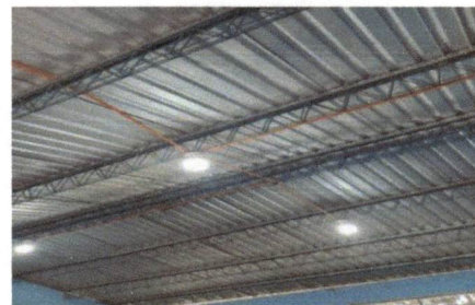
Foto 6: Reparación de sistema eléctrico: sustitución de lámparas, plafoneras, interruptores, tomacorrientes, sustitución de ducto eléctrico y reparación de cable eléctrico
