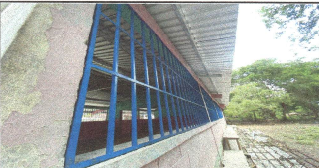
Foto 5: CAMBIO DE BALCONES NUEVOS, EN LAS DOS AULAS, DIRECCION Y BODEGA.
