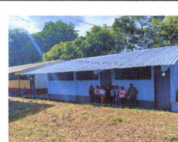
Foto 2: Sustitución de lámina, por lámina troquelada aluzinc calibre 26
