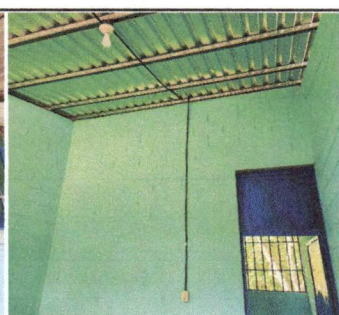
Foto 3: Sustitución de estructura de soporte de metal, por metal
