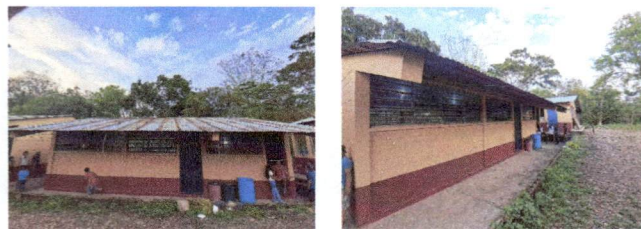
Foto 2 Sustitución de lámina, por lámina troquelada aluzinc calibre 26
