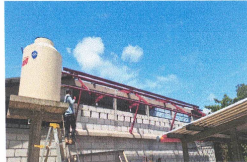
Foto 2: Sustitución de estructura de soporte de madera, por metal
