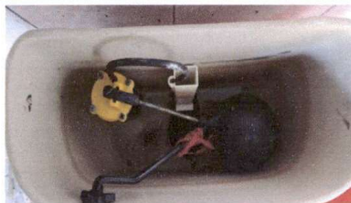
Foto 2: Sustitución de accesorios inodoro (contra llave, tubo de abasto y tanque)
