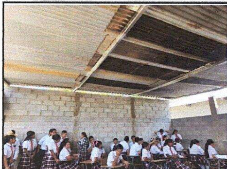
Foto: 3 Sustitución de lámina, por lámina troquelada aluzinc calibre 26
