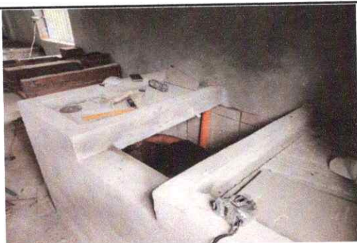
Foto 5: Sustitución de pila de cemento
