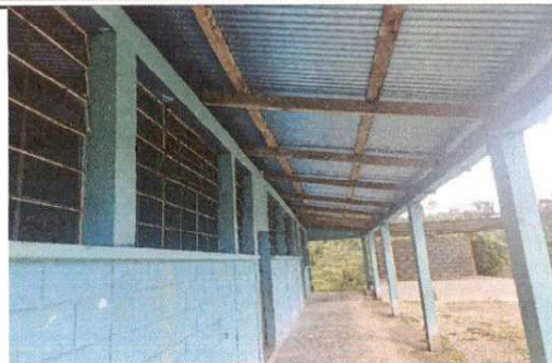
FOTO 2: SUSTITUCION DE ESTRUCTURA DE MADERA, POR METAL
