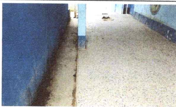
Foto 2: Reparación de cuneta de concreto + Rejilla
