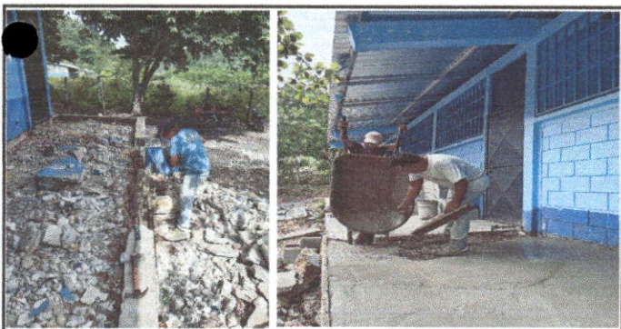
Foto 5. Reparación de banquetas de concreto
