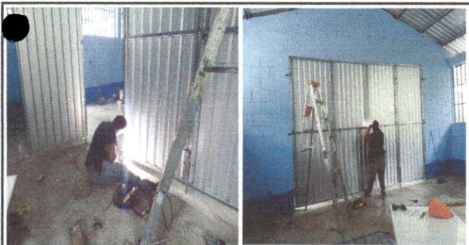
FOTO 5: División entre aulas
