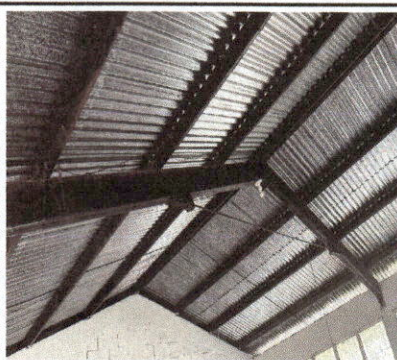
Foto 2: SUSTITUCIÓN DE LAMINA, POR LAMINA TROQUELADA ALUZINC CALIBRE 26
