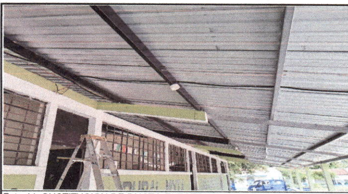
Foto 11: SUSTITUCION DE DUCTO ELECTRICO, SUSTITUCION DE INTERRUPTOR SIMPLE
