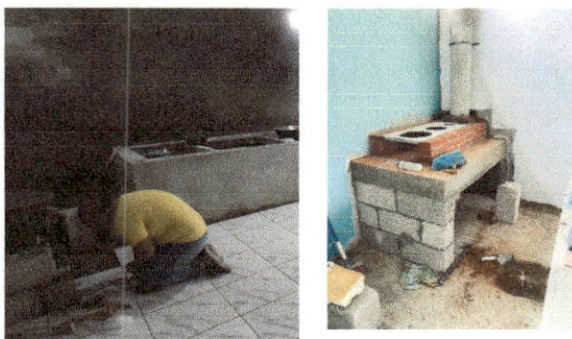
Foto: Sustitución de estufa rural (completa) incluye chimenea y plancha de metal
