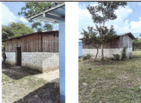
Foto 1: Sustitución de lámina, por lámina troquelada aluzinc calibre 26, Sustitución de estructura de soporte de madera, por metal
