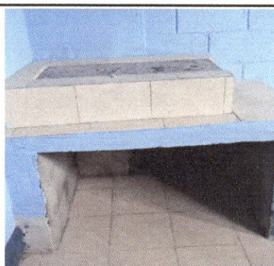
Foto 10: Instalación de azulejo en estufa rural
