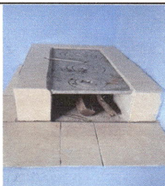
Foto 9: Sustrucción de estufa rural
