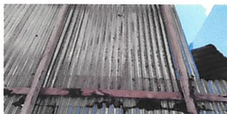
Foto 2: Sustitución de lámina, por lámina troquelada Aluzinc calibre 26
