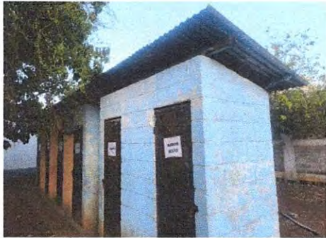
Foto 1: Sustrucion de lamina acanalada por lamina troquelada con aluzin calibre 26
