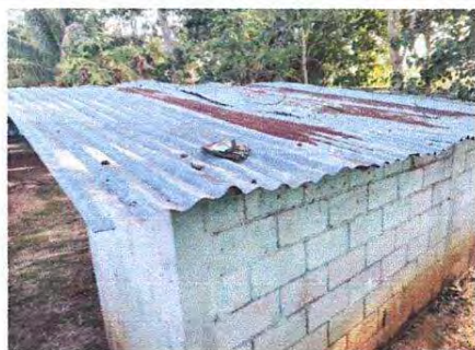
FOTO 13 SUSTITUCION DE LAMINA, POR LAMINA TROQUELADA ALUZINC CALIBRE 26
