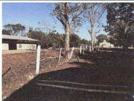
FOTO 3 - REPARACIÓN DE TUBO HG Y MALLA GALVANIZADA
