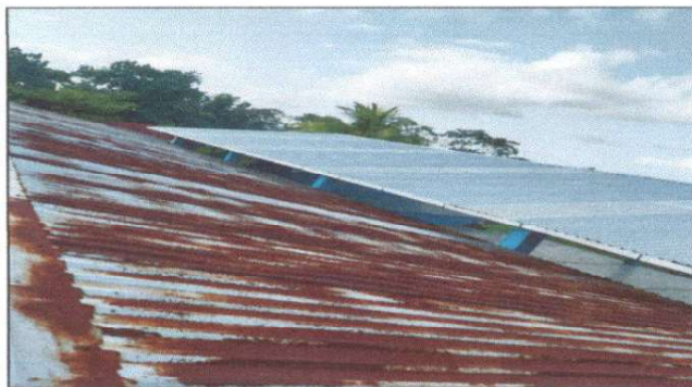
Foto 4: Sustrucción de lámina troquelada aluzinc
