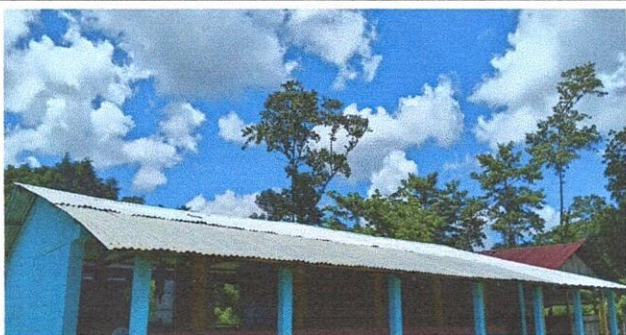
Foto 3: Sustitución de lámina, por lámina troquelada aluzinc calibre 26
