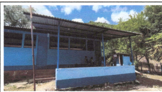
Foto 4: Sustitución de lámina, por lámina troquelada aluzinc calibre 26
