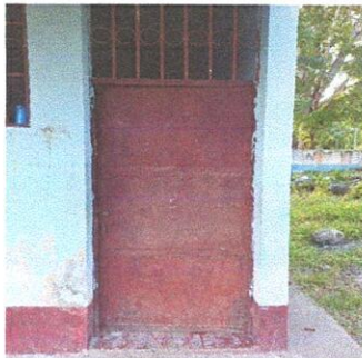
Foto 3: Mantenimiento a estructura (lijado, cambio de tubo, cepillado, sujeciones, aplicación de pintura)
