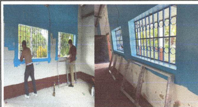
Foto 2: Fabricación e instalación de marcos de aluminio mil finish
