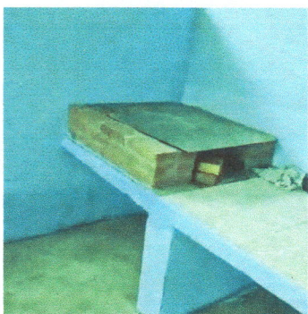
Foto 20: Sustitución de estufa rural (completa) incluye chimenea, 1 Plancha de hornillas y 1 plancha de metal lisa
