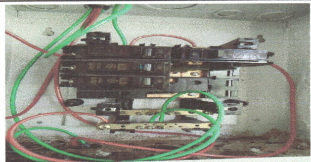
foto 12. sustitucion de flipones 2
