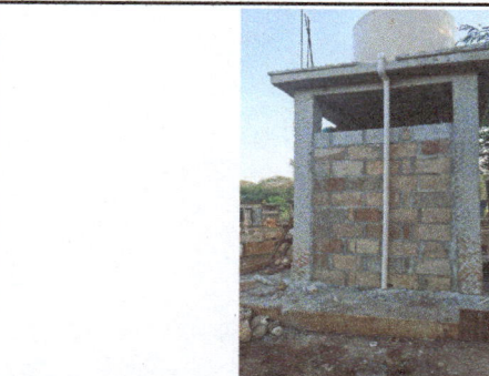
Foto 5: Sustitución de puertas de metal de servicios sanitarios
