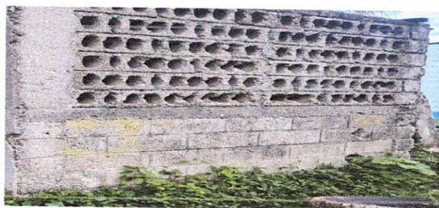
FOTO 13. REPARACION DE MURO DE CONTENCIÓN
