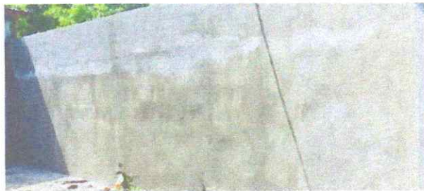
Foto 2: Reparación de muro perimetral de block con tubo hg y malla galvanizada, soleras intermedias y columnas.
