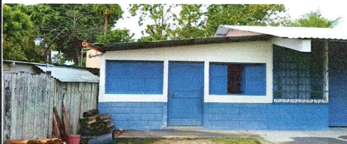
Foto 1: No.1 Sustitución de lámina, por lámina troquelada aluzinc calibre 26, Sustitución de estructura de soporte de madera, por metal
