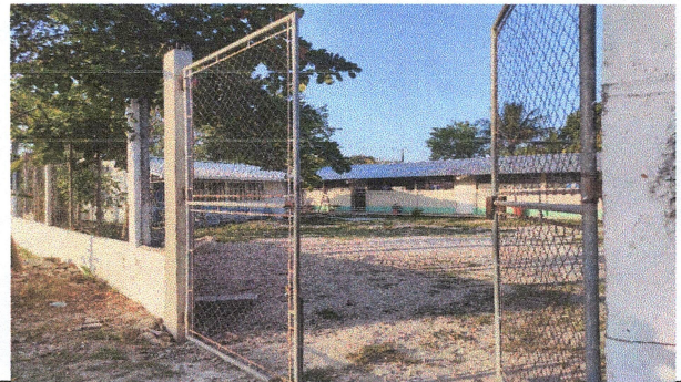
Foto 4: REPARACIÓN DE TUBO HG Y MALLA GALVANIZADA, Los trabajos consisten en la desinstalación de la malla perimetral y tubo HG en su totalidad, e intalar tubo HG y malla galvanizada nueva.
