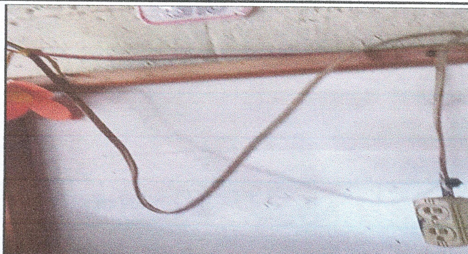
Foto 2: INSTALACIONES DE UNIDADES DE FUERZA TOMACORRIENTES INCLUYE CABLE ELECTRICO. Los trabajos consisten en la instalación de 21 tomacorrientes en los diferentes ambientes de la escuela con su respectiva distribución de nuevos circuitos individualizados por aula y sus respectivas cajas de flipones, así como la instalación de cableado nuevo para estos.
