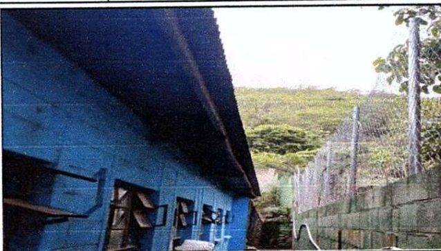
Foto 8: INSTALACIÓN DE TUBOS DE PVC DE 4" PARA CANALES Y BAJADA DE AGUAS PLUVIALES
