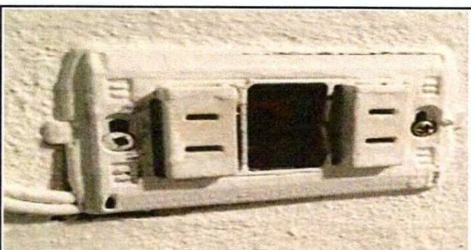
Foto 5: Sustitucion toma corrientes
