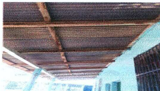
Foto 2:MODULO ARE CORREDOR Estructura de madera dañada y sustituir, lámina mal estado .
