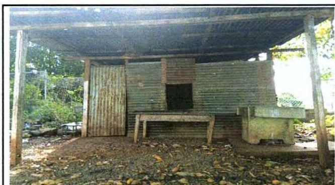
Foto 3: Piso de torta de concreto en mal estado en área interna y externa de cocina a mejorar con piso de cerámico en área interna y torta de concreto en área frontal.
