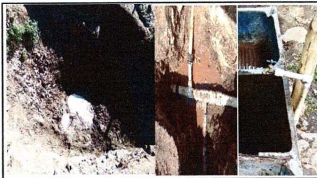
Foto 4: Reparación de red de drenaje y agua potable
