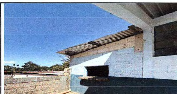
Foto 4: Mejoramiento de sillar a pestaña y dintel para ventana en cocina.
