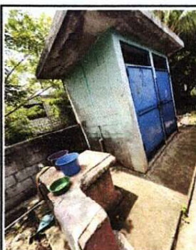
Foto 4: Área de Baños, remozamiento de puertas, sustitución de pared de block, sustitución de puerta, sustitución de tazas de inodoro para niño y adulto, lavamanos, remozamiento de instalación de agua potable.
