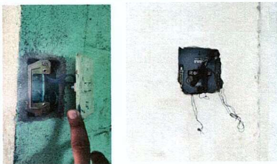
Foto 5: INSTALACION DE UNIDADES DE LUZ
