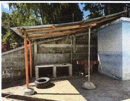
Foto1: MODULO DE COCINA NECESIDADES: CERRAMIENTO, CUBIERTA DE LAMINA, CONSTRUCCIÓN DE ESTUFA RURAL Y MUEBLE BAJO FUNDIDO, CONTRAPISO, PISO, PILA, PUERTA, VENTANAS.
