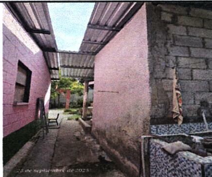
FOTO 2: REPARACIÓN DE REPELLO Y CERNIDO EN PAREDES
