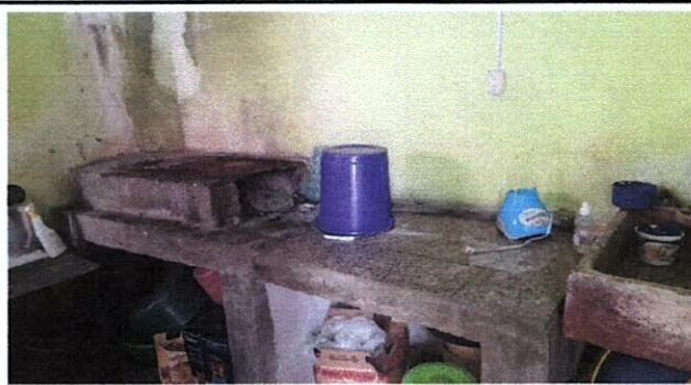
FOTO 4: REPARACIÓN DE COCINA (MANTENIMIENTO A ESTUFA RURAL Y SUS AGREGADOS)
